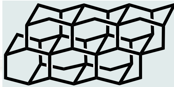
Diamondoid 2-3nm
